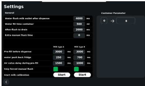
3.4.5 Milk module settings
